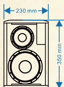
主视图
